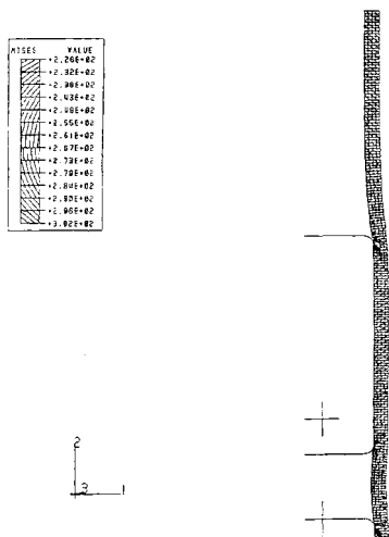
Slika 7: Von Misesova ekvivalentna napetost v matrici pri 12,5% deformaciji (MISES (N/mm 2 ))
